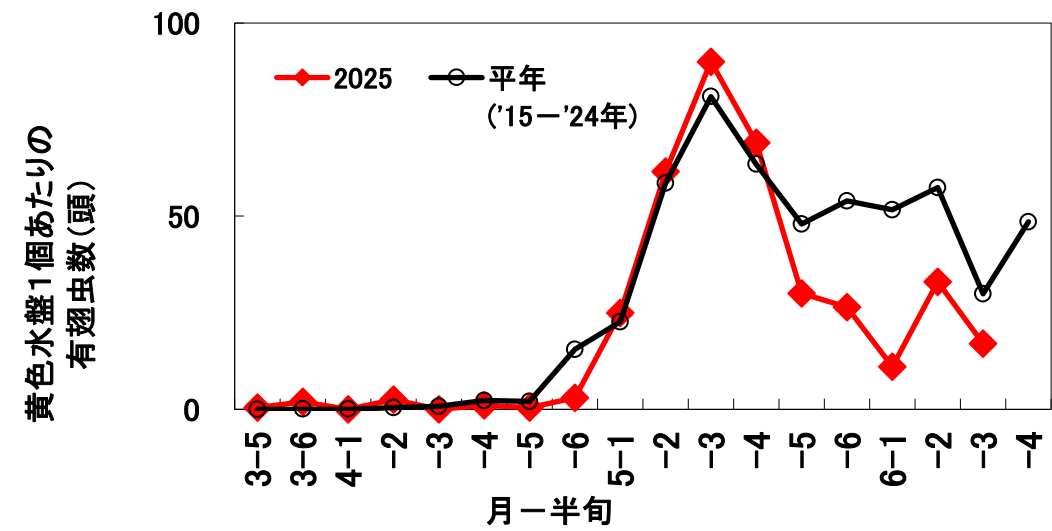
図 アブラムシ有翅虫の飛来消長
